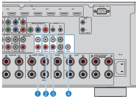
Аппарат (вид сзади)
