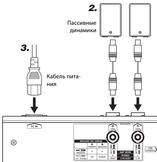
Задняя панель (См. стр. 14.)
