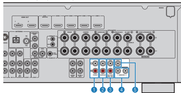
Данный аппарат (вид сзади)
