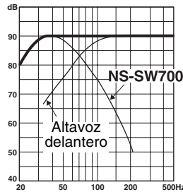
Gráfico de respuesta de frecuencia*
