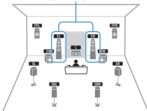
Двухканальное усиление
