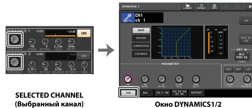
Окно DYNAMICS1/2
