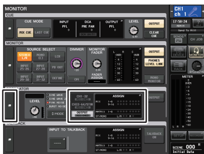
Экран MONITOR
