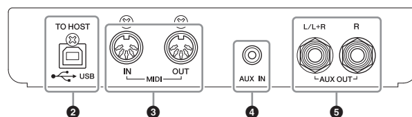
Панель разъемов (в правой нижней части клавиатуры)
