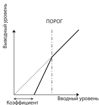
Характеристики I/O (KNEE=hard, OUT GAIN=0.0dB)
