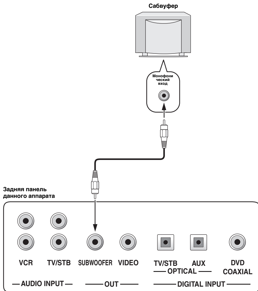
Кабель сабвуфера
