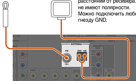
Комнатная FM-антенна
