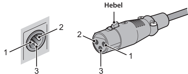
XLR-Buchse (männlich)
